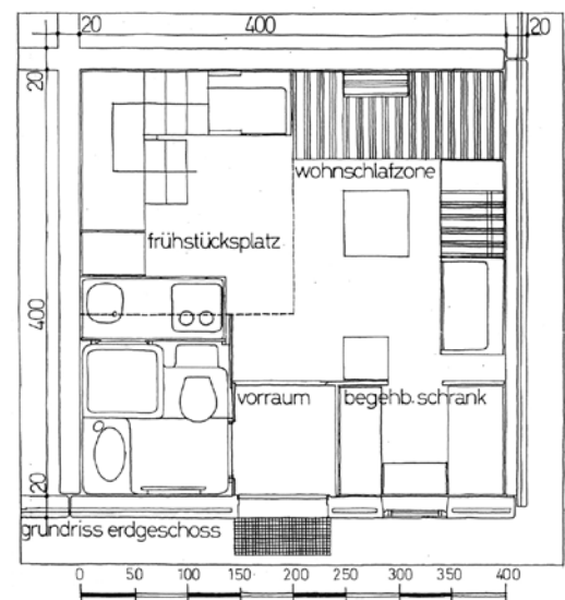
Grundriss Olympiabungalows München
